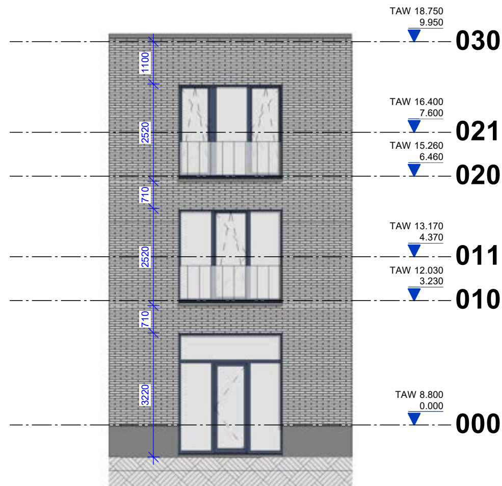
Schaal: 1 : 100 Voorgevel
