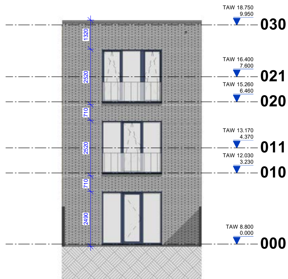
Schaal: 1 : 100 Achtergevel
